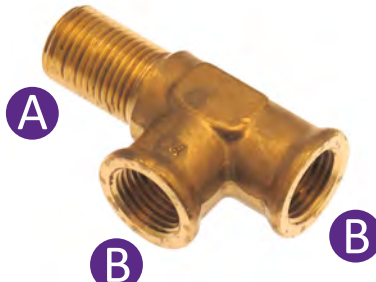
Side Stud Tee
